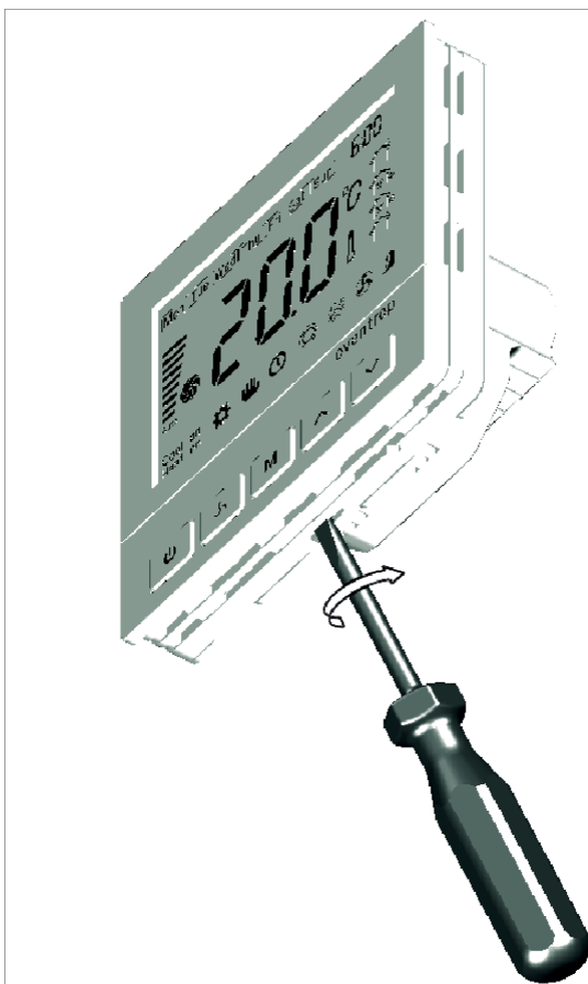
Рис. 4: Отсоединение панели управления
