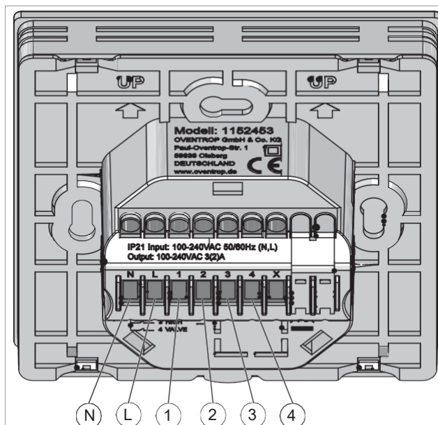
Рис. 5: Распределение клемм
