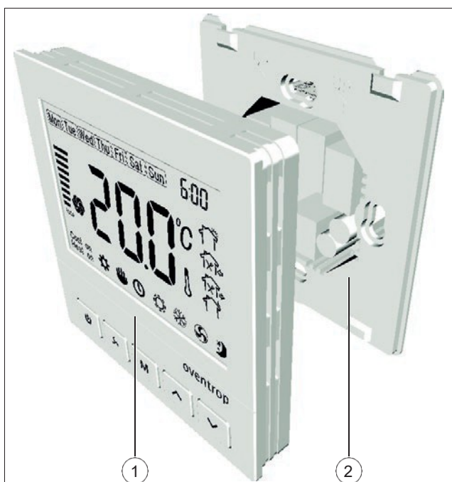
Рис. 1: Конструкция
