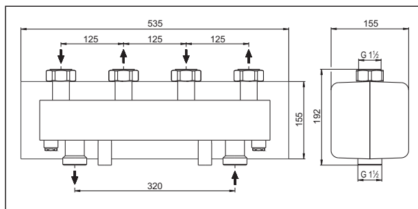
Размеры „HydroFixx“ DN 25, на 2 контура
