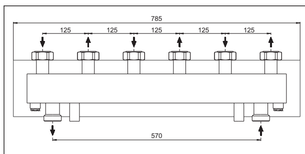
Размеры „HydroFixx“ DN 25, на 3 контура
