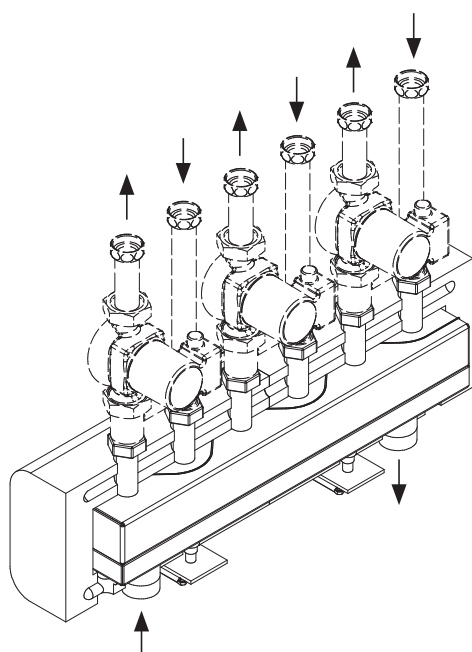
Для 3 / 5 / 7 ... отопительных контуров
