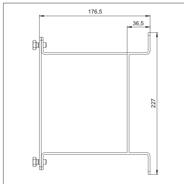
Размеры настенного крепежа
