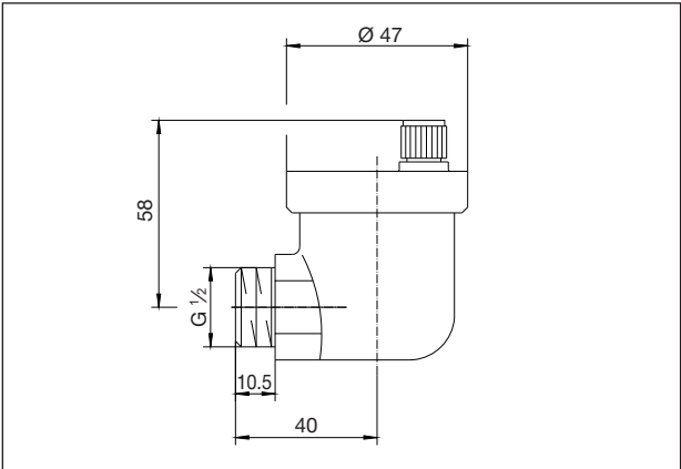
Размеры артикул № 108 84 04
