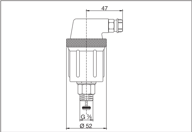
Размеры артикул № 108 82 03
