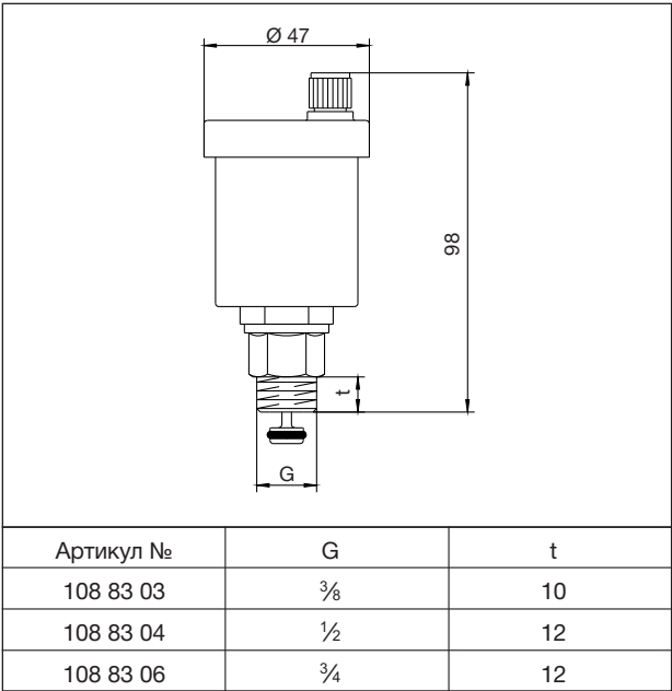
Размеры артикул № 108 83 03-06
