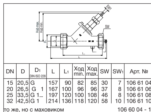
Размеры вентил для слива
