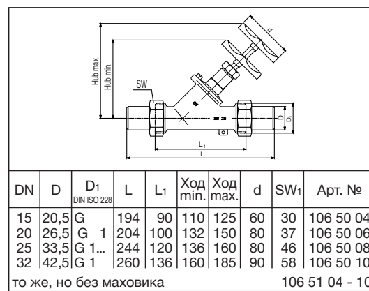
Размеры запорного вентил
