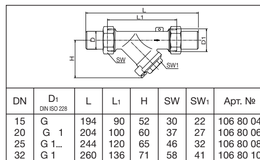
Размеры фильтра
