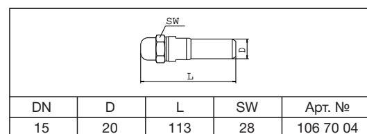
Размеры воздухоотводчика
